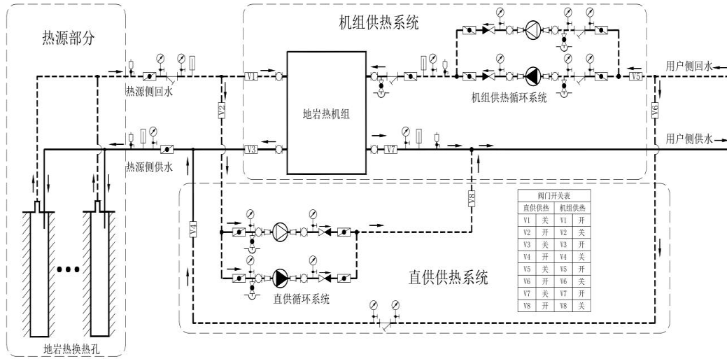
图 5 系统运行原理图
