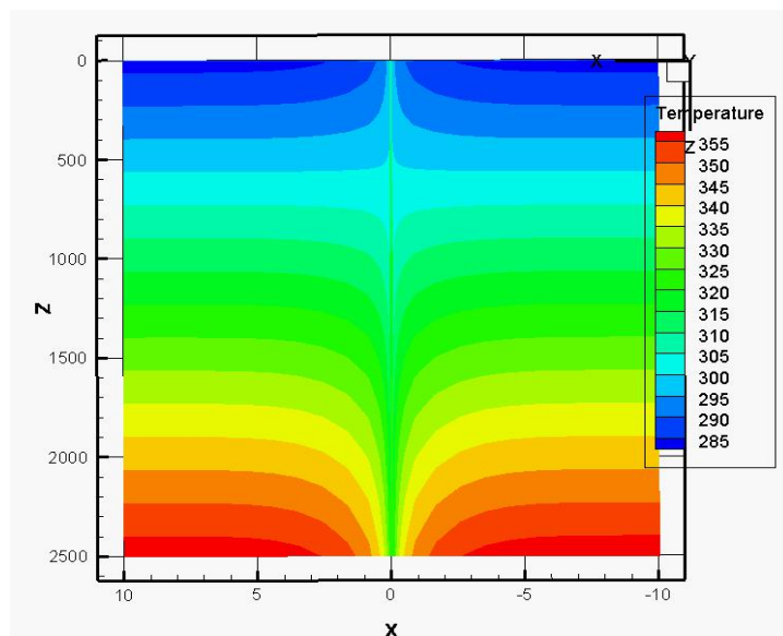
图 3 热影响半径
