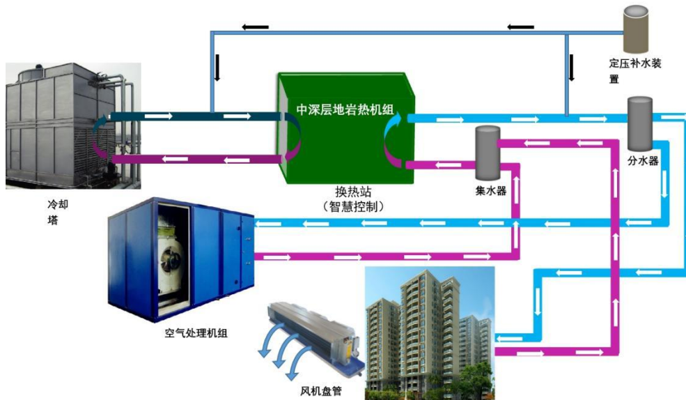
图2 系统制冷示意图
