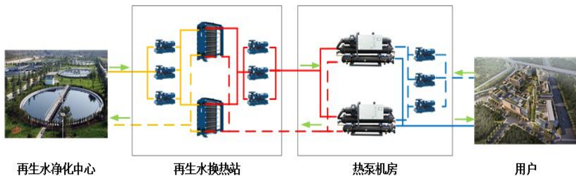
图2 再生水源热泵系统示意图
