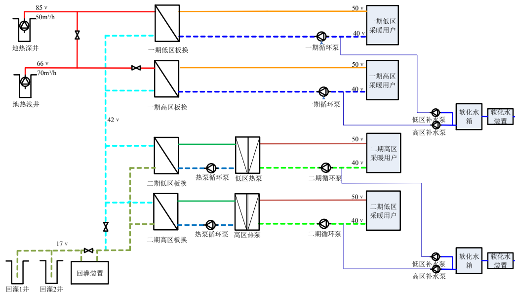
图 1 项目供暖工艺流程图
