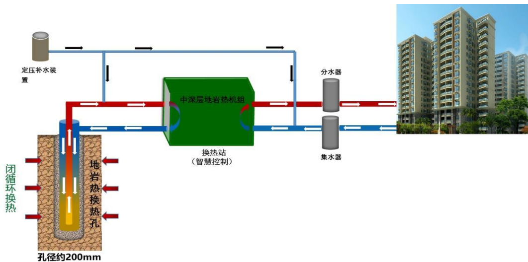
图1 系统供热示意图
