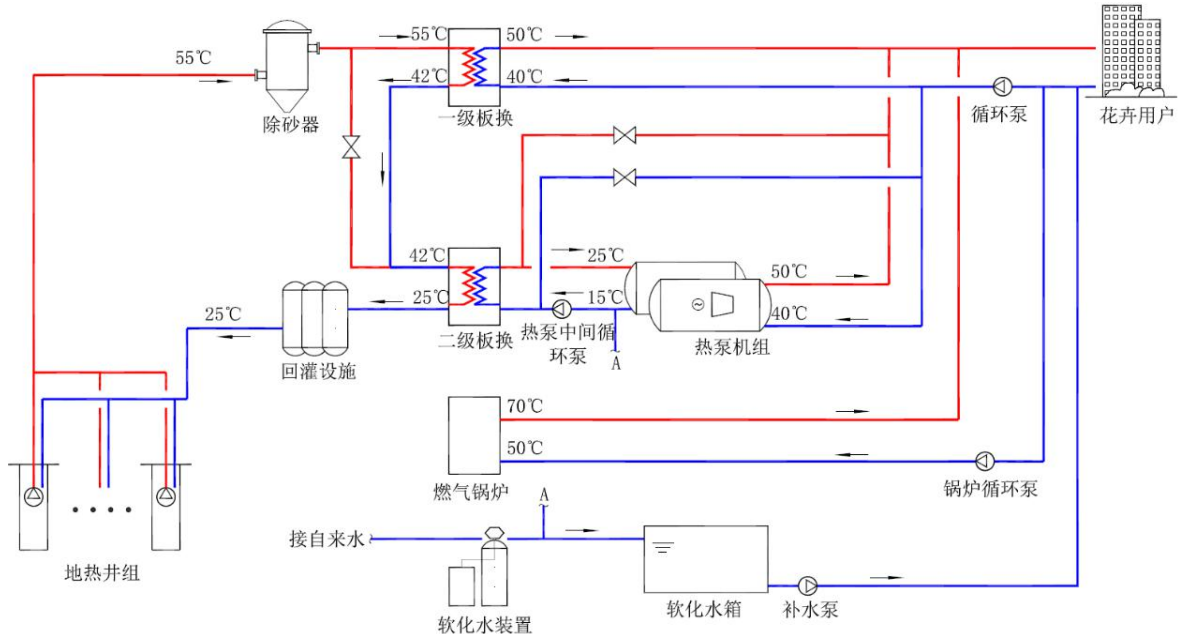
图 1 地热供热系统工艺流程图
